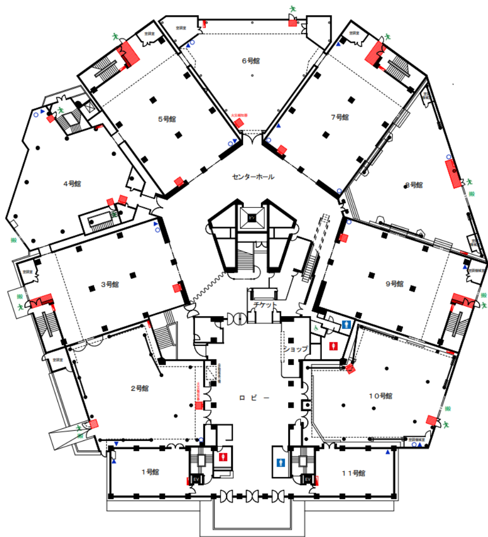
展示・イベントホール全体配置図
